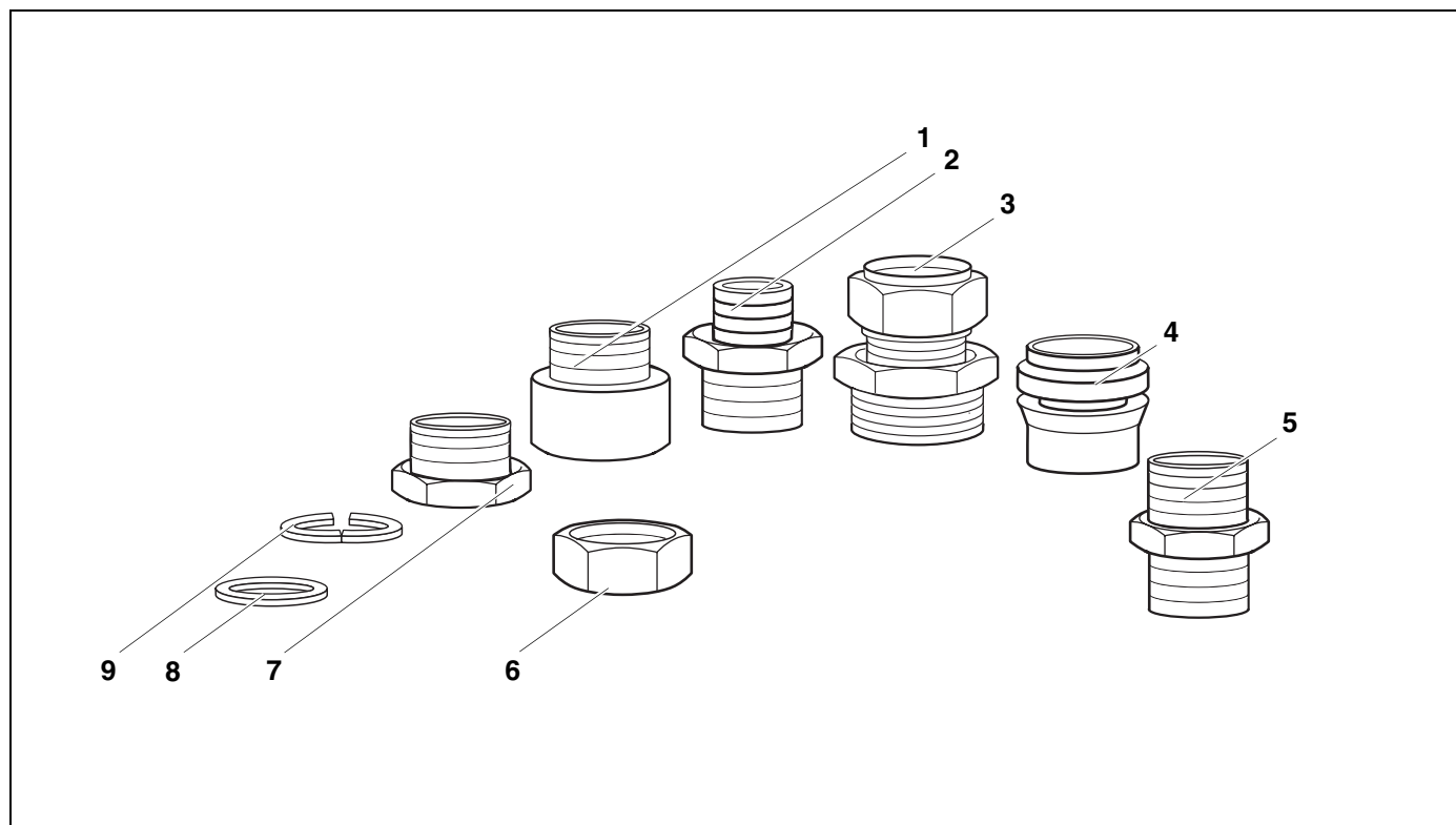
Fig. 1 Set di collegamento Twin Tube DN 20
