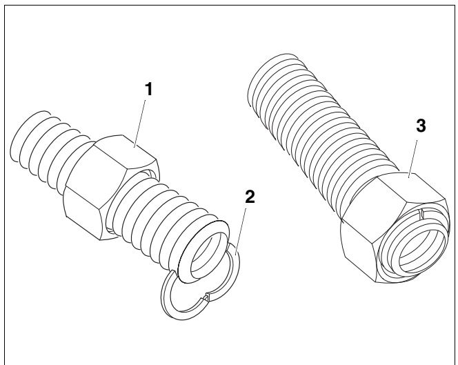
Fig. 2 Montare la rondella di bloccaggio
