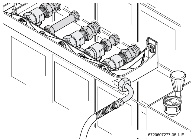
Fig. 5 Messa in pressione dei circuiti idraulici mediante apposita pompa (max 15 bar).
