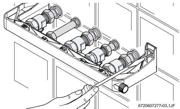
Fig. 3 Fissaggio della dima in plastica
