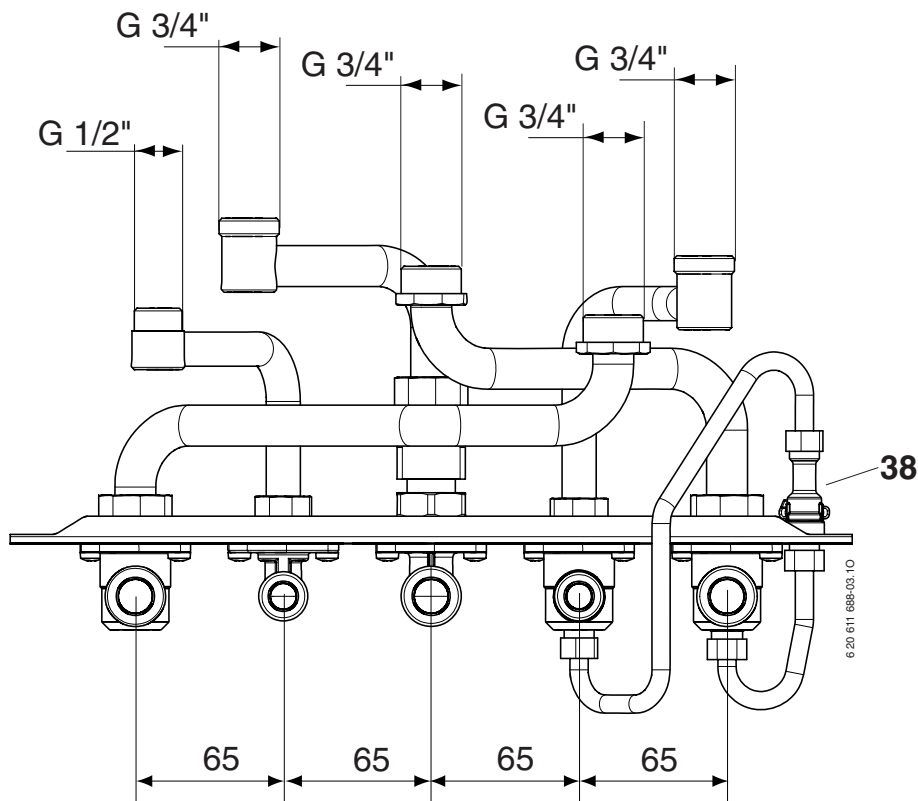
Fig. 3 Piastra di allacciamento e raccordi di collegamento all'impianto (DOS GA 6R)
