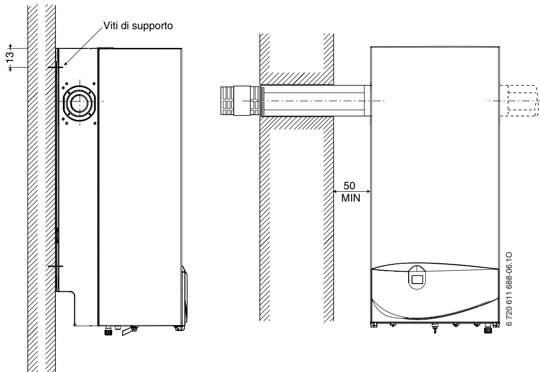
Fig. 2 Aspirazione/scarico laterale (DX o SX)
