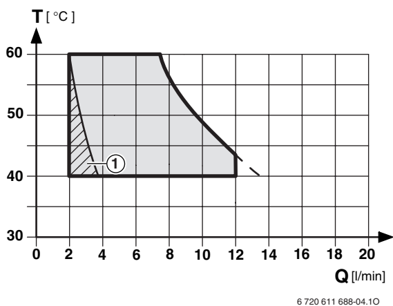
Fig. 27 Diagramma indicativo riferito con ingresso a +15°C
