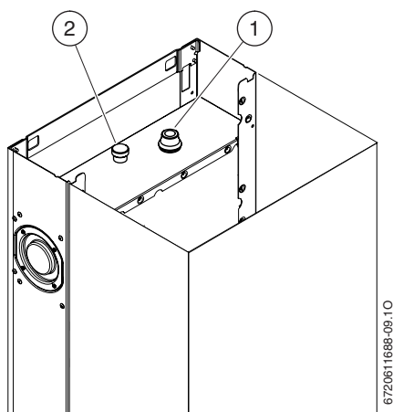
Fig. 64 Analisi di combustione
