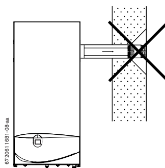
Fig. 12 Montaggio non autorizzato
