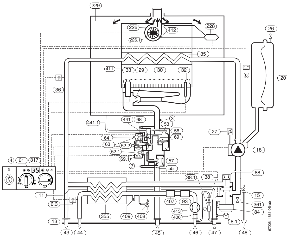
Fig. 4 Schema di funzionamento
