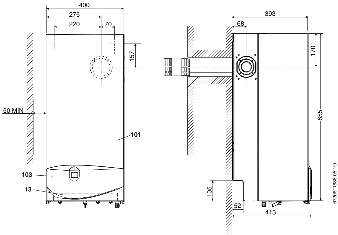
Fig. 1 Aspirazione scarico posteriore
